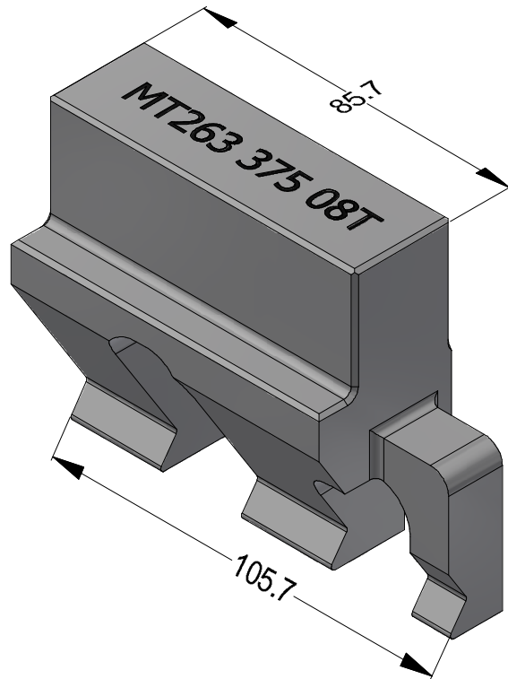
Sandvik MT263 375 08T
